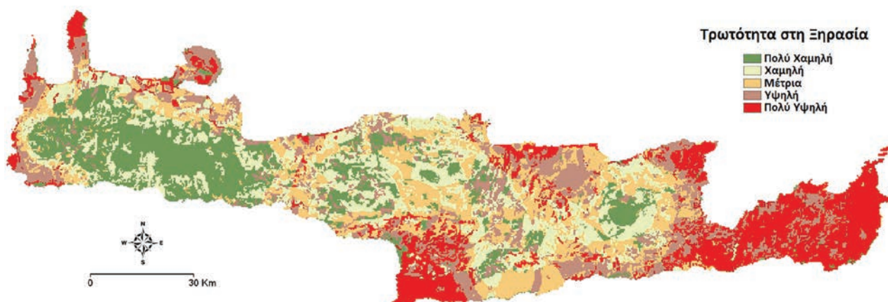
Χωρική κατανομή των επιπέδων τρωτότητας στην Ξηρασία για το Υδατικό Διαμέρισμα Κρήτης.
